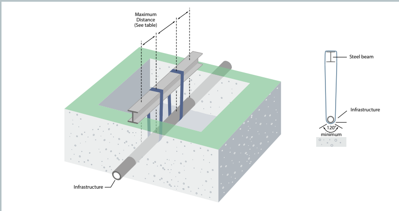
Figure 7 - Overhead Support (Exemple for Énergir et Enbridge Gaz Québec).
